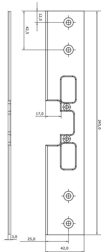
Monteringsstolpe 917W
