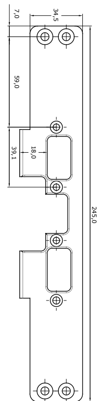
Monteringsstolpe 942
