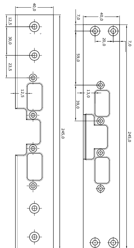
Monteringsstolpe 965W
