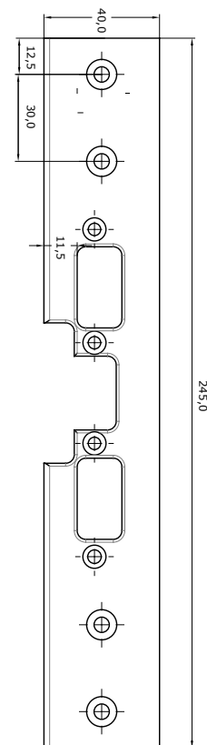
Monteringsstolpe 965W
