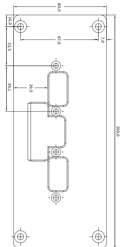
Monteringsstolpe 959
