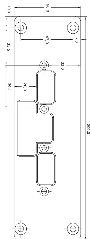
Monteringsstolpe 957
