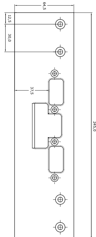
Monteringsstolpe 975-S
