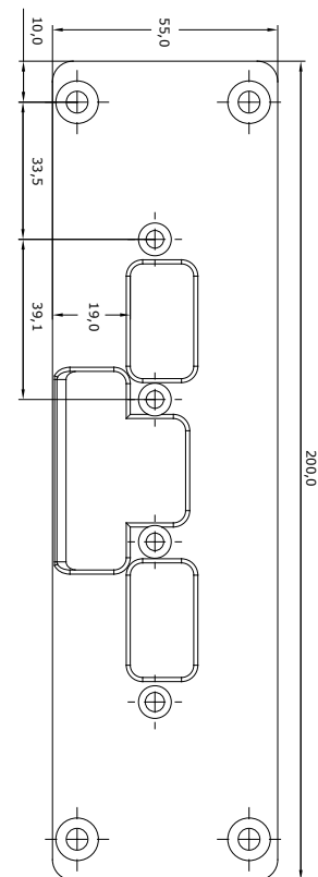
Monteringsstolpe 956
