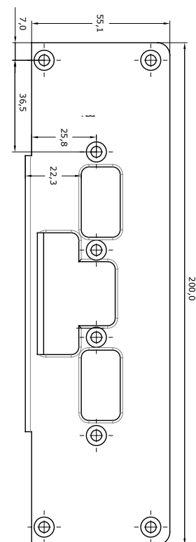
Monteringsstolpe 9487-10
