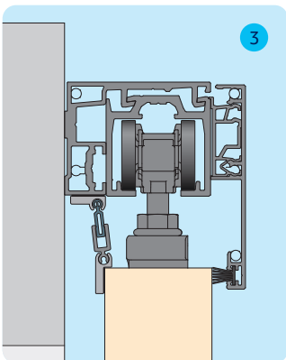
3. Wandmontage mit Variante A-B innen geklebt
