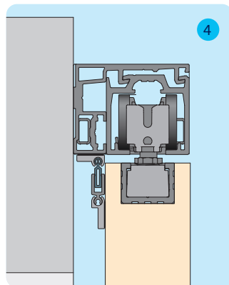
4. Wandmontage mit Variante A-B aussen geklebt
