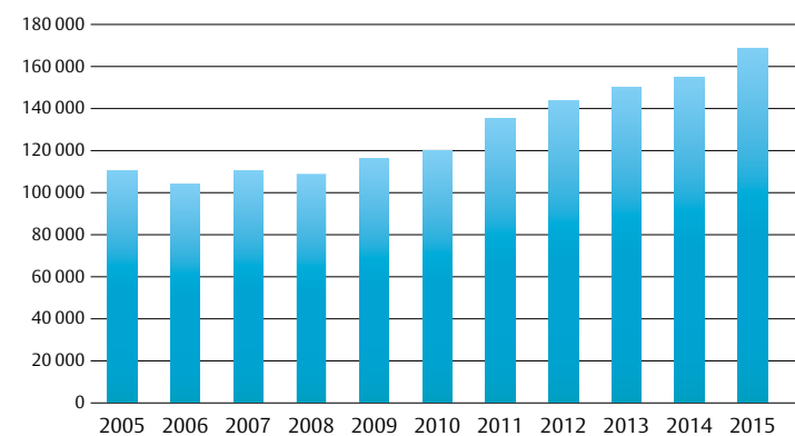
Einbruchstatistik Deutschland
