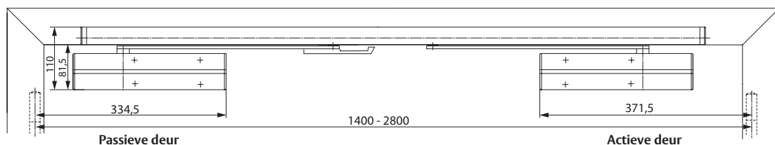
2 - Deurbladmontage niet-scharnierzijde
